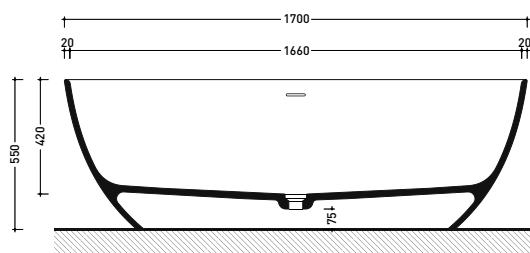
sezione longitudinale / section
